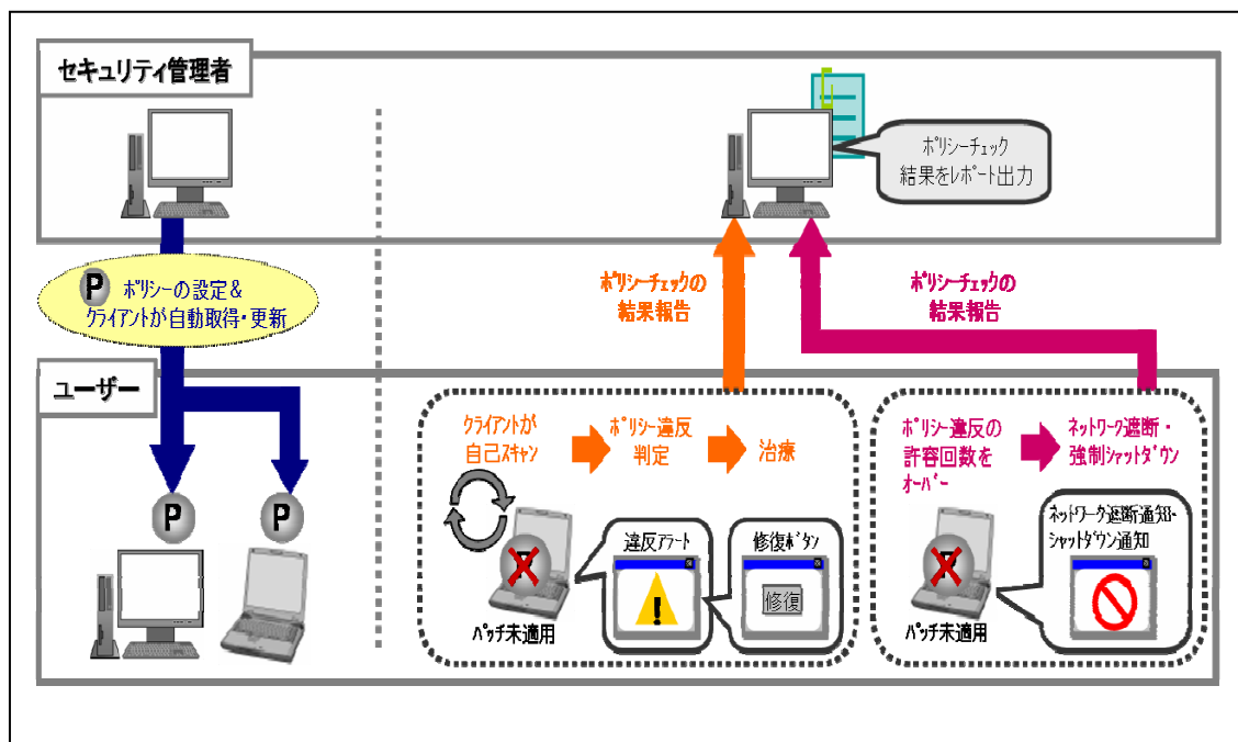
「AdminITy Ver4.2 システムイメージ図」
